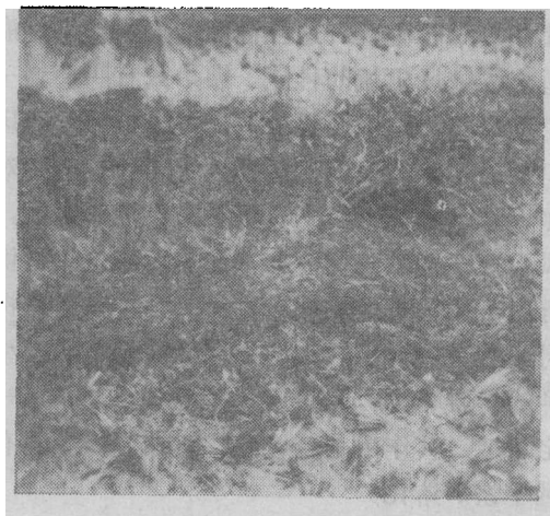
图八 铁炉村炒炉遗址的结铁
